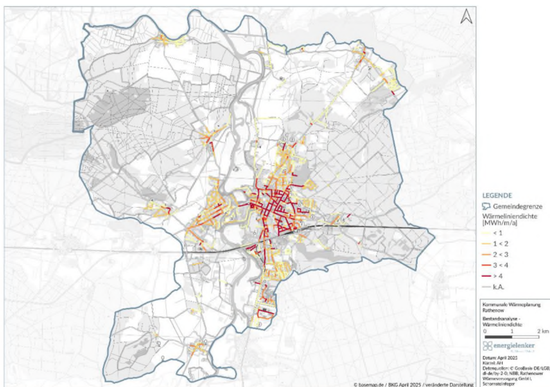
Abbildung 1 Wärmelinien-dichte Rathenows im Jahr 2023
